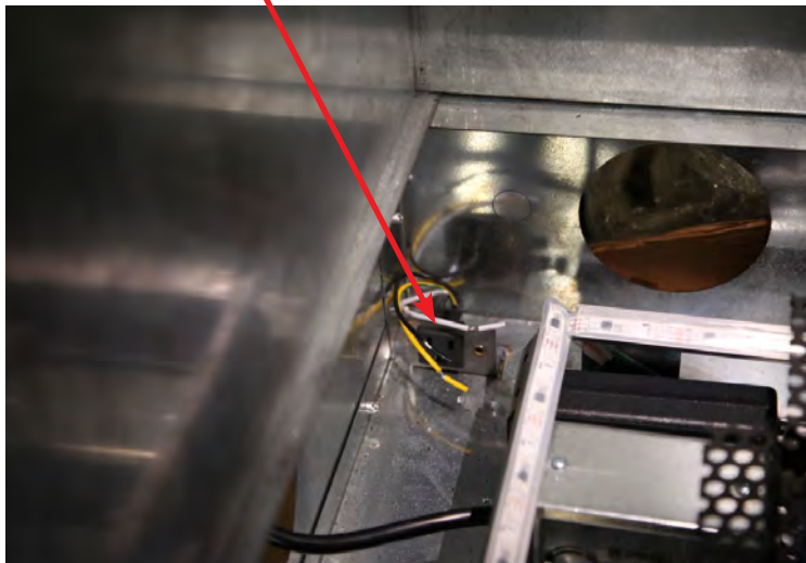
Conduit clamp
